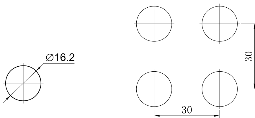
单件安装开孔尺寸
