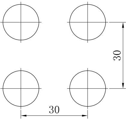
多件组合安装开孔尺寸
